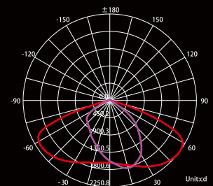
C Plane [50%MaxAng.][10%MaxAng.]
